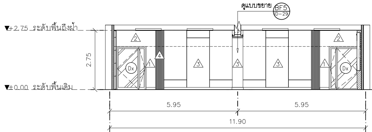
แบบขยายรูปตัดภายใน มาตราส่วน 1:100 A ID-14
