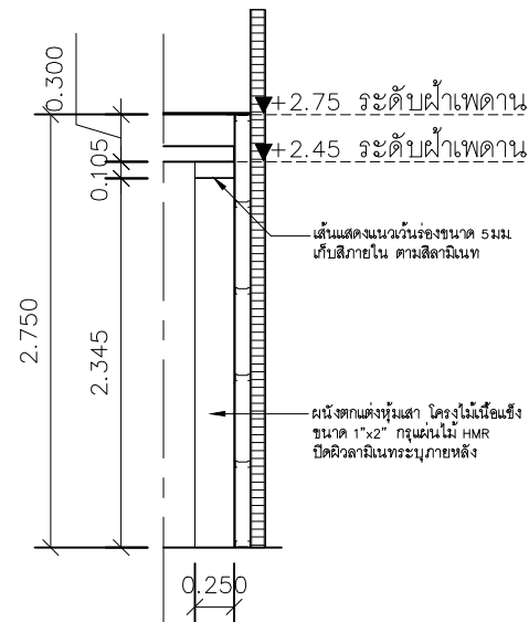
ห้องเรียน 2404-2504 แบบขยายรูปด้านข้าง BW2
