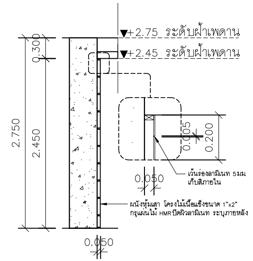
ห้องเรียน 2404-2504 แบบขยายรูปตัด 15
