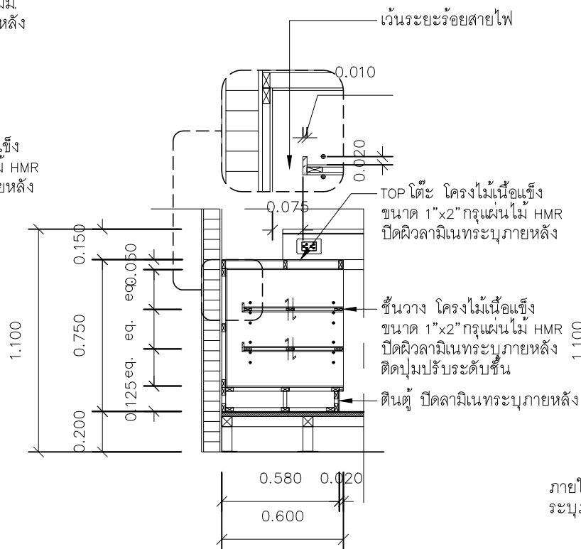
ห้องเรียน 2508(ศรีตรัง) แบบขยายรูปตัด 5
