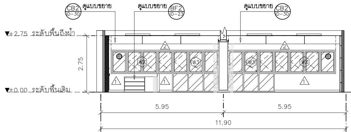
แบบขยายรูปตัดภายใน มาตราส่วน 1:100 C ID-15
