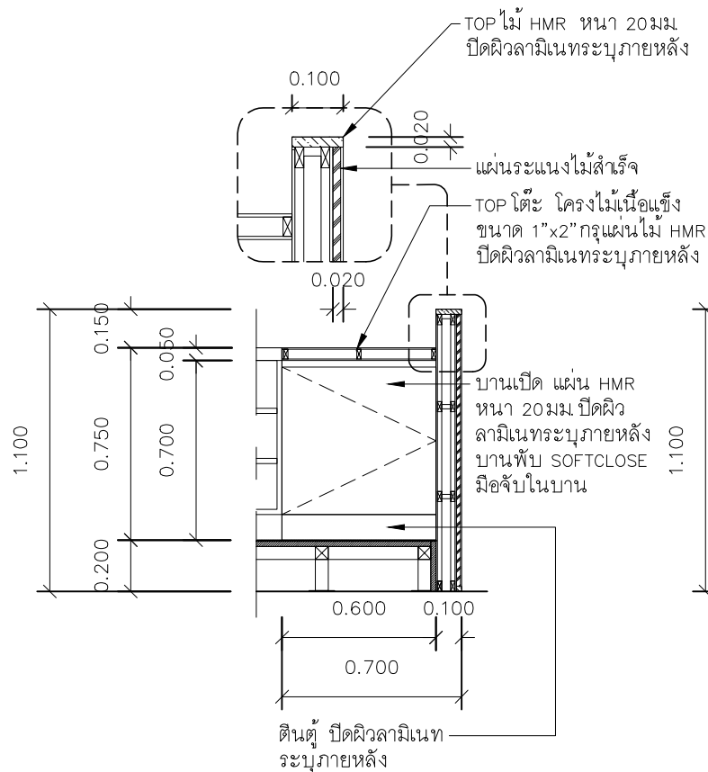
ห้องเรียน 2508(ศรีตรัง) แบบขยายรูปตัด 4
