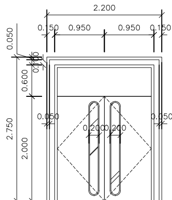
Ⓓ ประตูไม้ตกแต่งบานเปิดคู่ (ห้องเรียน 2508 ครีตริง)
