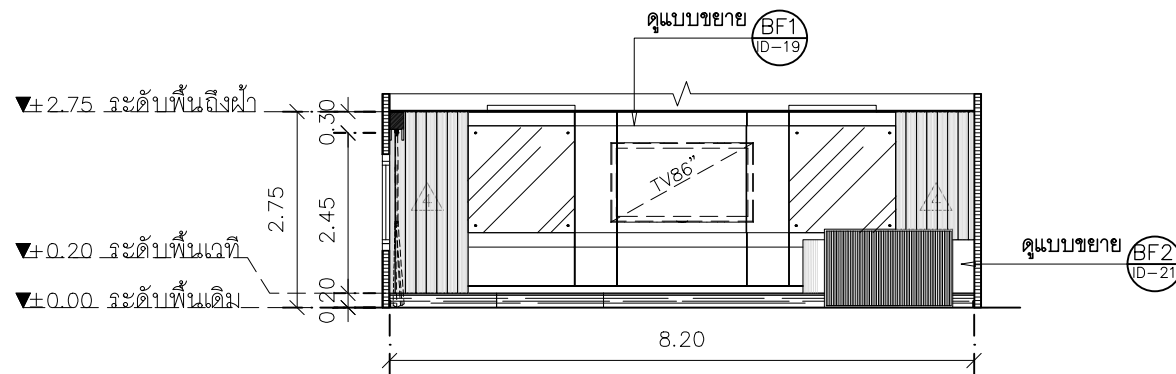
แบบขยายรูปตัดภายใน มาตราส่วน 1:100
