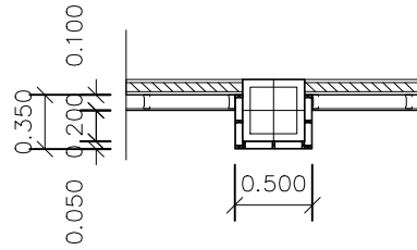
ห้องเรียน 2404-2504 แบบแปลน BW2
