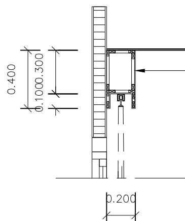
ห้องเรียน 2508(คริตร์ง) แบบขยายรูปตัด 16
