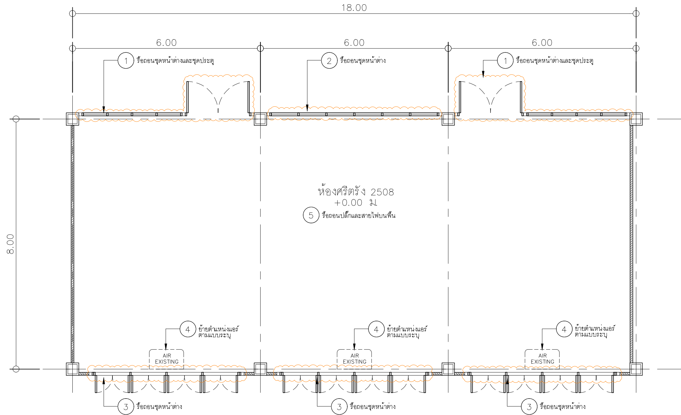
ห้องเรียน 2508(ศรีตรัง) แปลนปรับอากาศ มาตราส่วน 1:100
