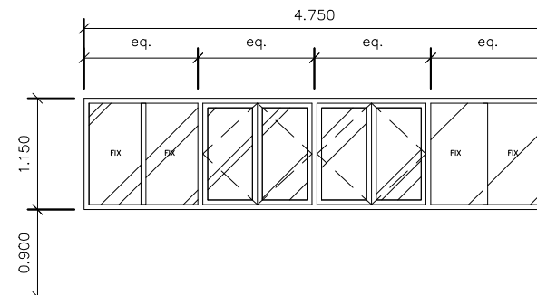
Ⓦ1 หน้าต่างอลูมิเนียมบานเปิดคู่ พร้อมบานปิด (ห้องเรียน 2508 ครีตริง)
