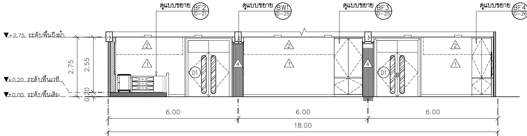
แบบขยายรูปตัดภายใน มาตราส่วน 1:100
