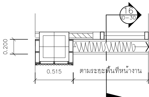
ห้องเรียน 2508(คริตร์ง) แบบแปลน CB1
