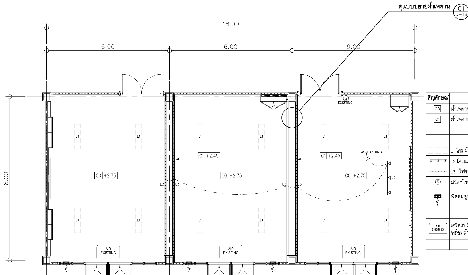
ห้องเรียน 2508(ครีตรัง) แปลนฝ้าเพดานและดวงโคม มาตราส่วน 1:100
